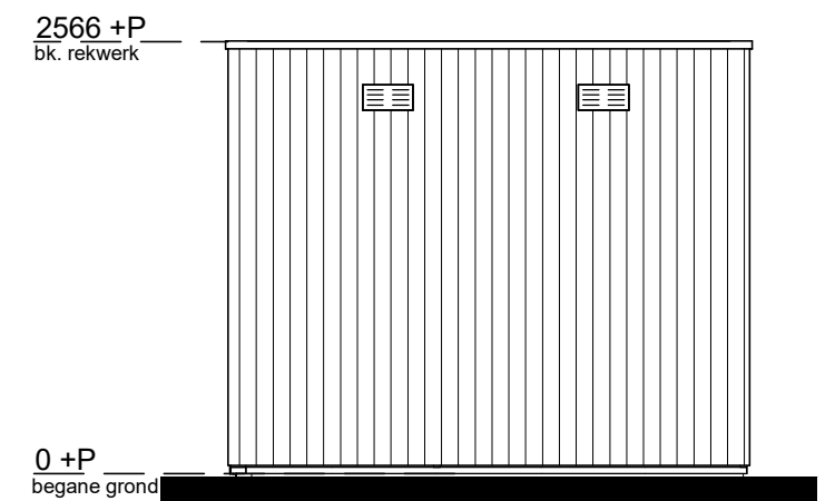
achtergevel
