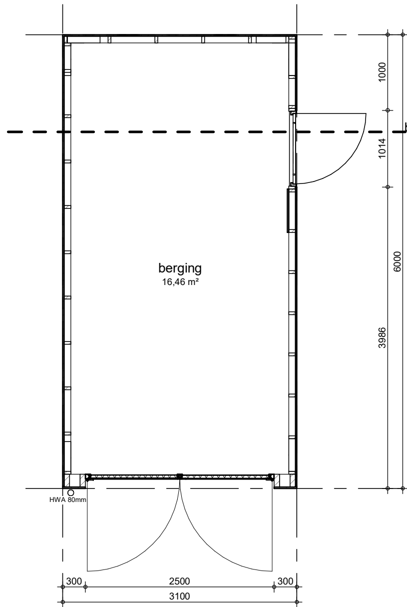
begane grond
