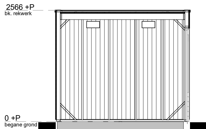
doorsnede A
