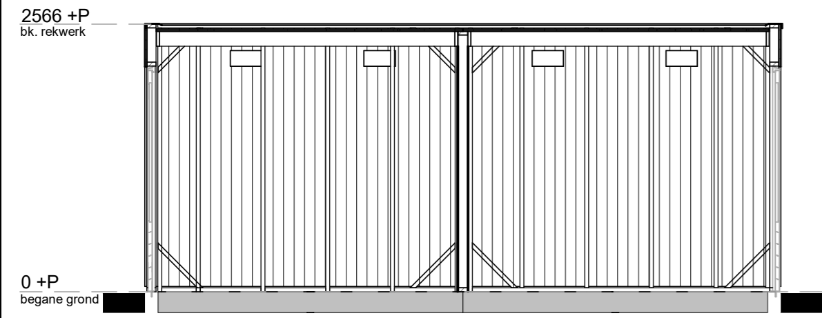
doorsnede A
