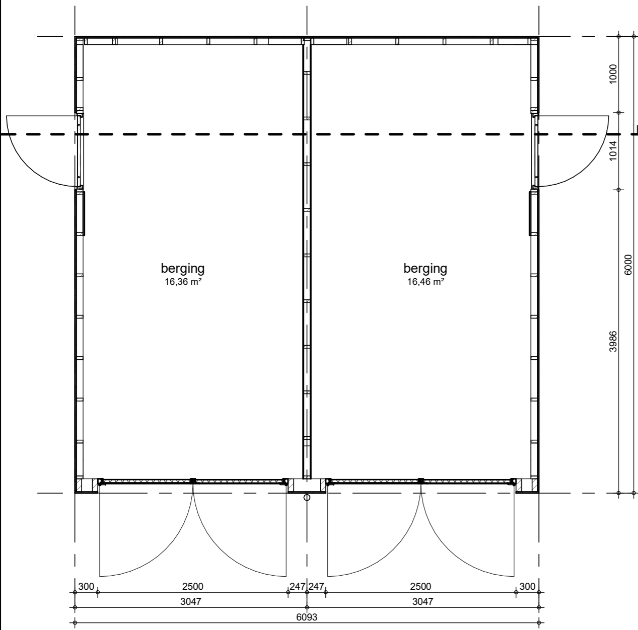
begane grond
